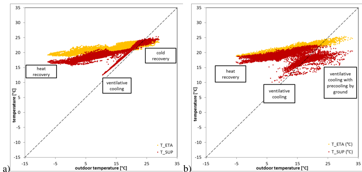
Afbeelding 2: Retourtemperatuur (geel) en toevoertemperatuur (rood) afhankelijk van buitentemperatuur voor veldtest DE03 (a) en veldtest “Nulwoning” (b).
