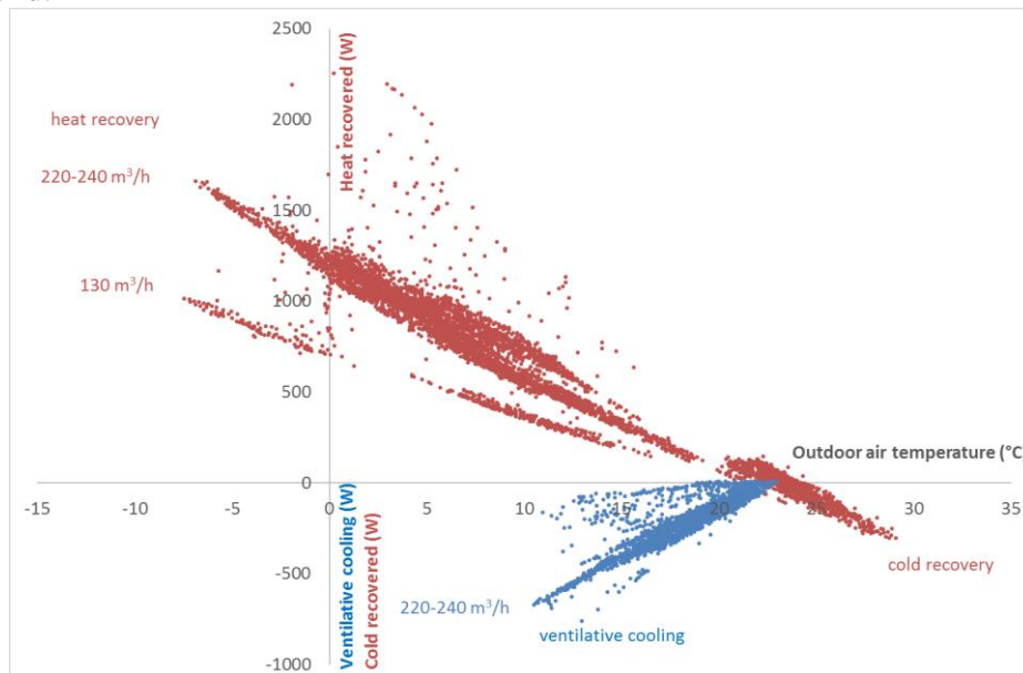
Afbeelding 3: Teruggewonnen warmte (rode stippen boven de horizontale as), ventilatiekoeling (blauwe stippen) en teruggewonnen koude (rode stippen onder de horizontale as) voor veldtest DE03.
