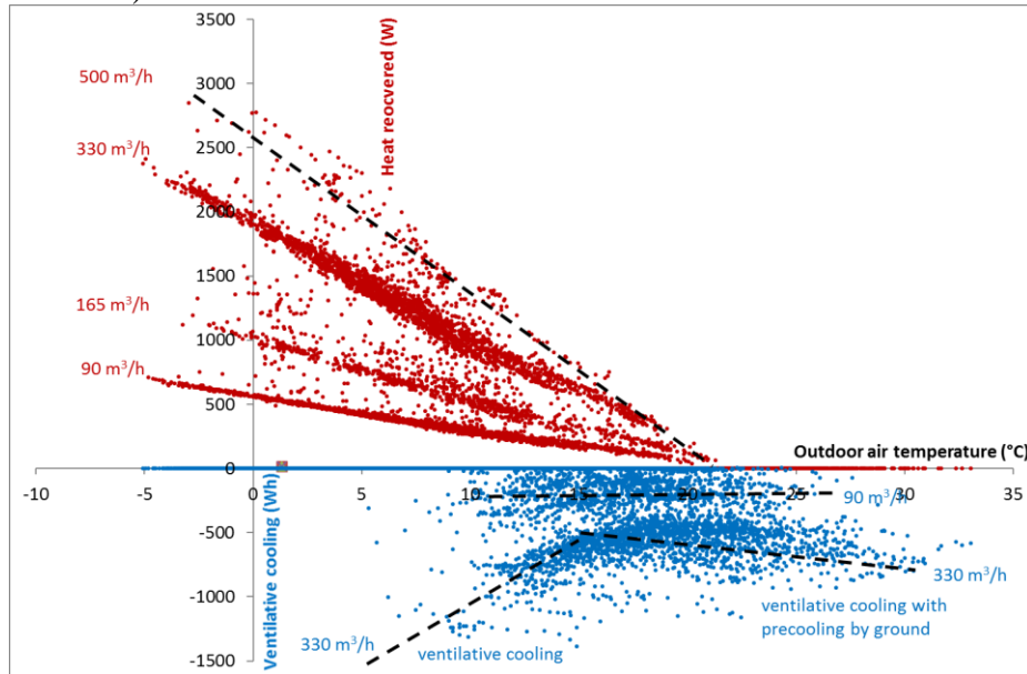
Afbeelding 4: Teruggewonnen warmte (rode stippen) en ventilatiekoeling (blauwe stippen) als functie van de buitentemperatuur voor veldtest “Nulwoning”.
